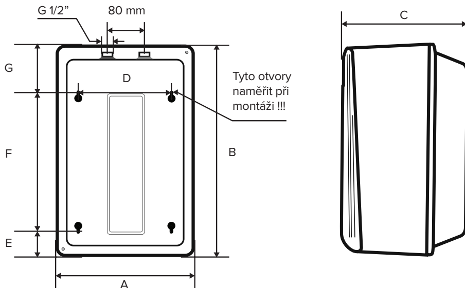
obr. 3: popis rozměrů pro montáž.
