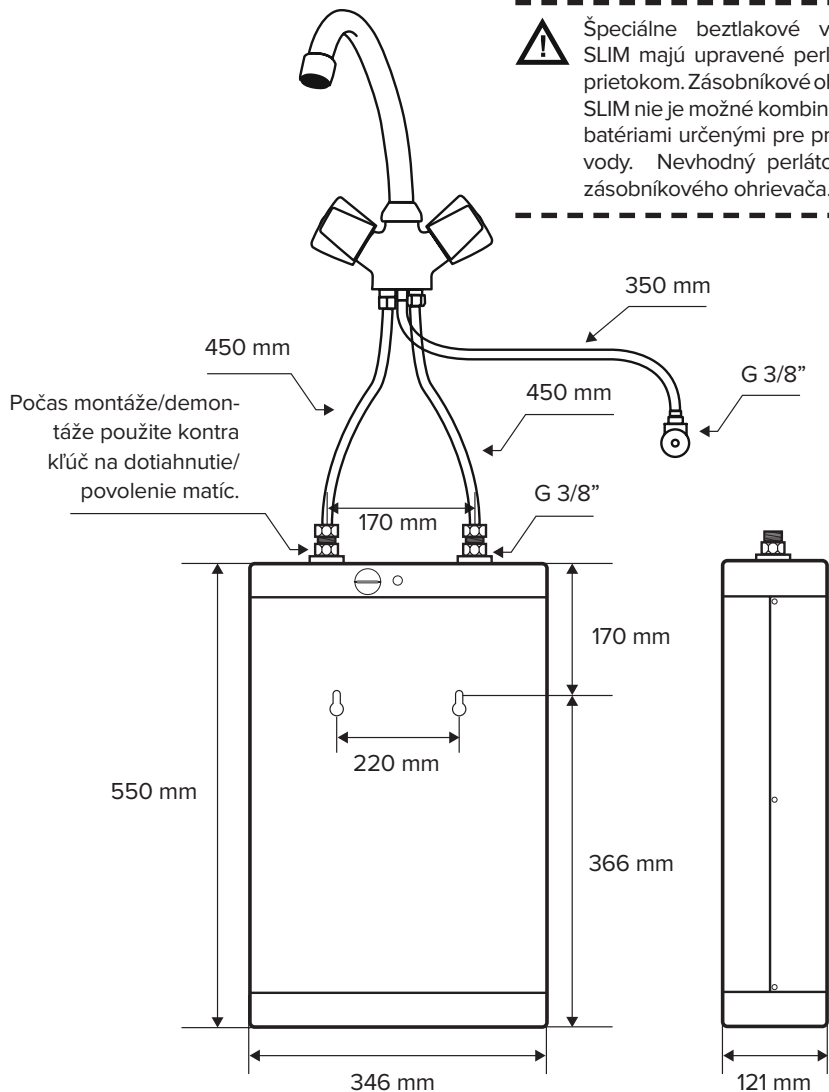
obr. 3: popis rozmerov pre montáž.
